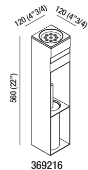
Elemento combinato in acciaio inox: Multipurpose element in stainless steel:
